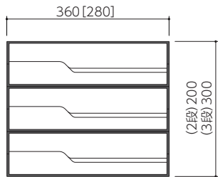
(投入口側)
