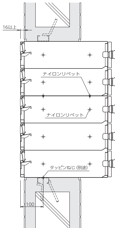
●納まり図
